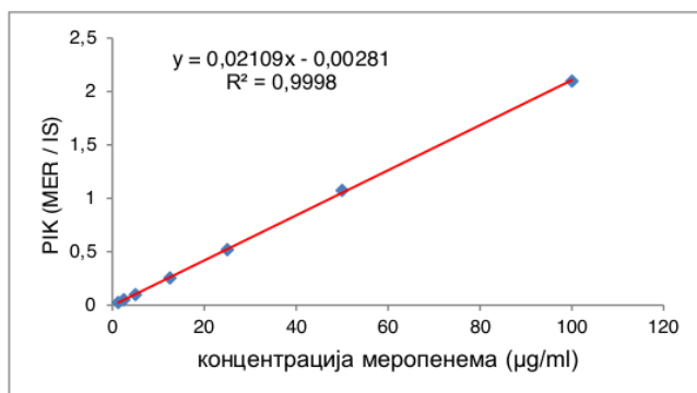
Слика 3. Калибрациона крива за одређивање меропенема
