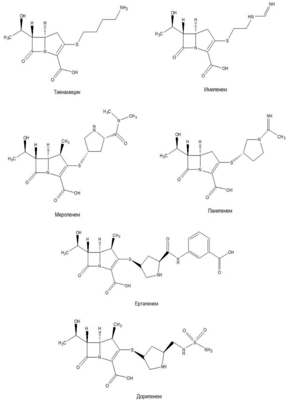
Слика 1. Хемијске структуре појединих представника карбапенема
