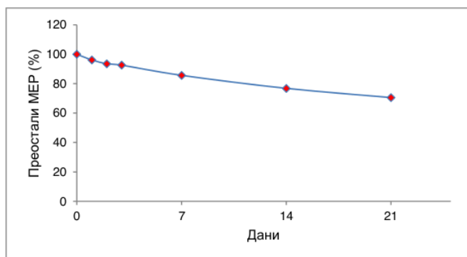
Слика 4. Стабилност меропенема у узорку плазме пацијента (44,2 µg/mL) без стабилизатора током три недеље на -20 °C
